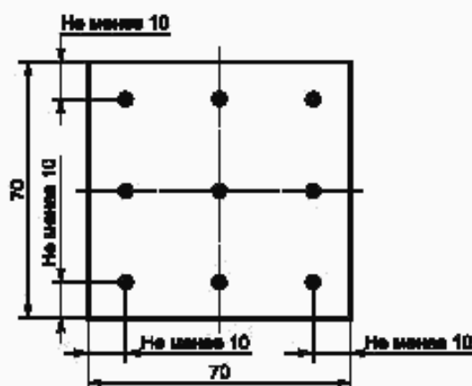
Рисунок 1 — Точки измерения толщины образца
