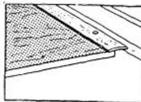
Рис. 6. Укладка металлической накладки на стыке двух видов покрытий
