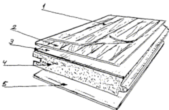
Рис. 2. Строение ламинированного напольного покрытия - доска ламинат-паркета:
