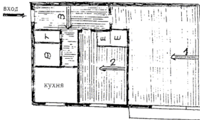
Рис. 3. Схема укладки досок ламинат-паркета:
