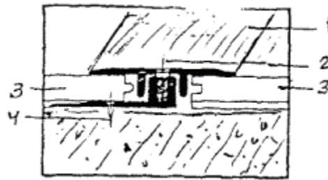
Рис. 4. Установка расширительного соединения:
