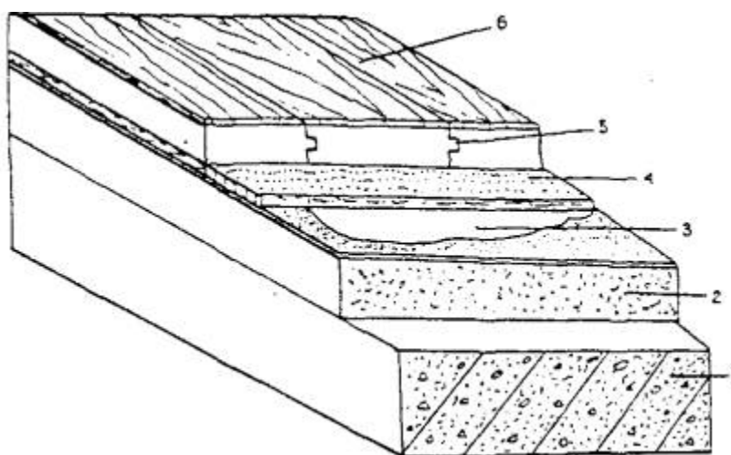
Рис. 1. Конструкция пола с покрытием из ламинат-паркета:
